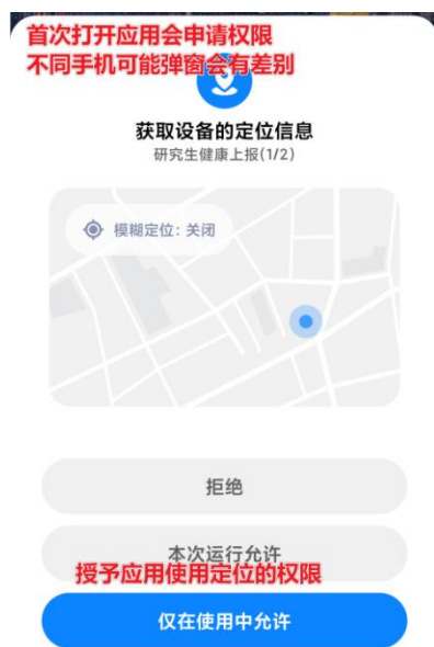
图 4 安卓版本
