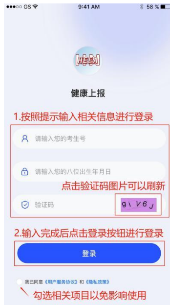
图 3 登录页面
